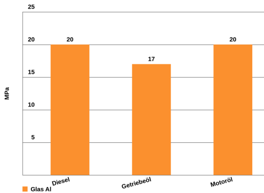
Druckscherfestigkeit nach Medienlagerung für 1000 h, DELO-Norm 5
